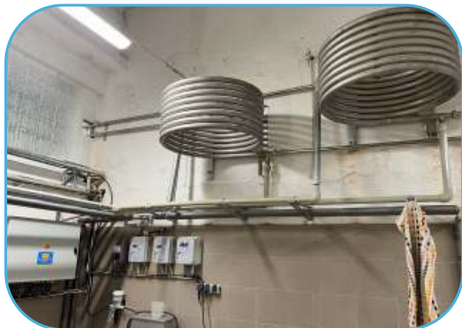
trubkový předchladič mléka
