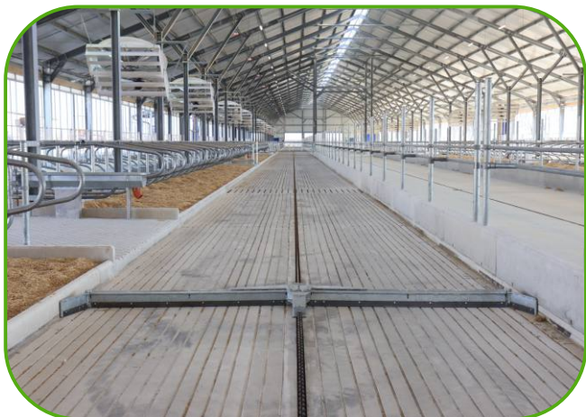
řetězová shrnovací lopata na odklíz kejdy, systém DELTA II
