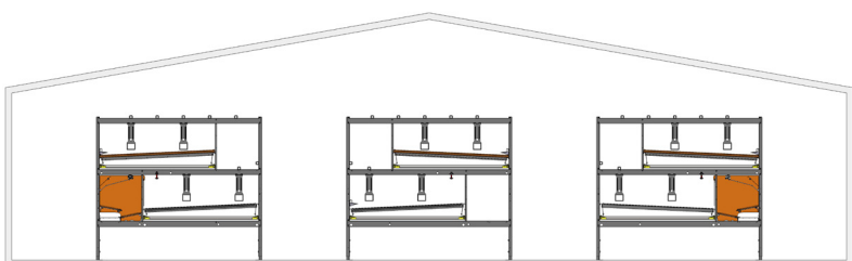
Compact 2+1 s 1 hnízdem, bez hnízd a s 1 hnízdem
